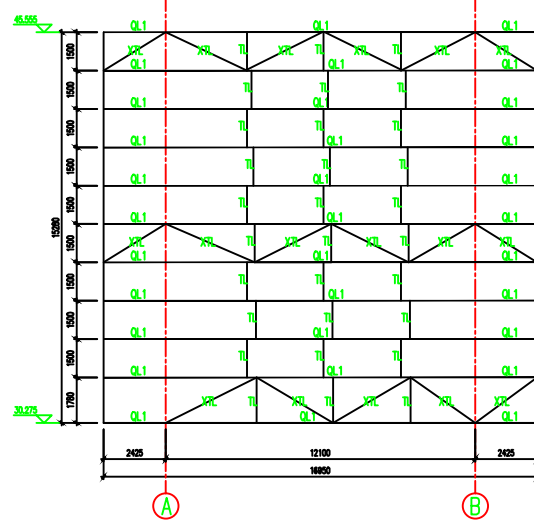
2-2 標条布置图
