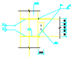
梁柱连接节点
